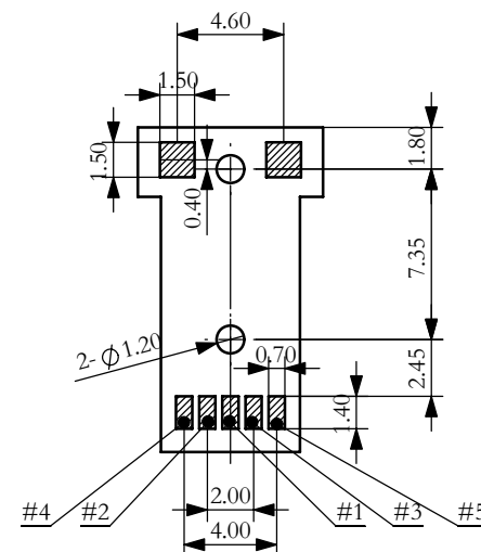
PCB布局参考图
