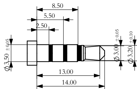
3.5标准插头
